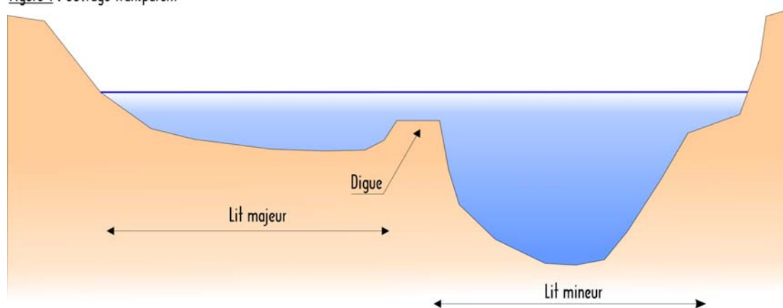
Figure 1 : Ouvrage transparent
